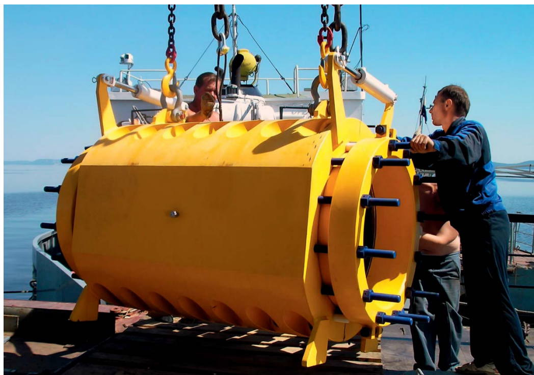
Подготовка муфты для ремонта подводного перехода трубопровода
